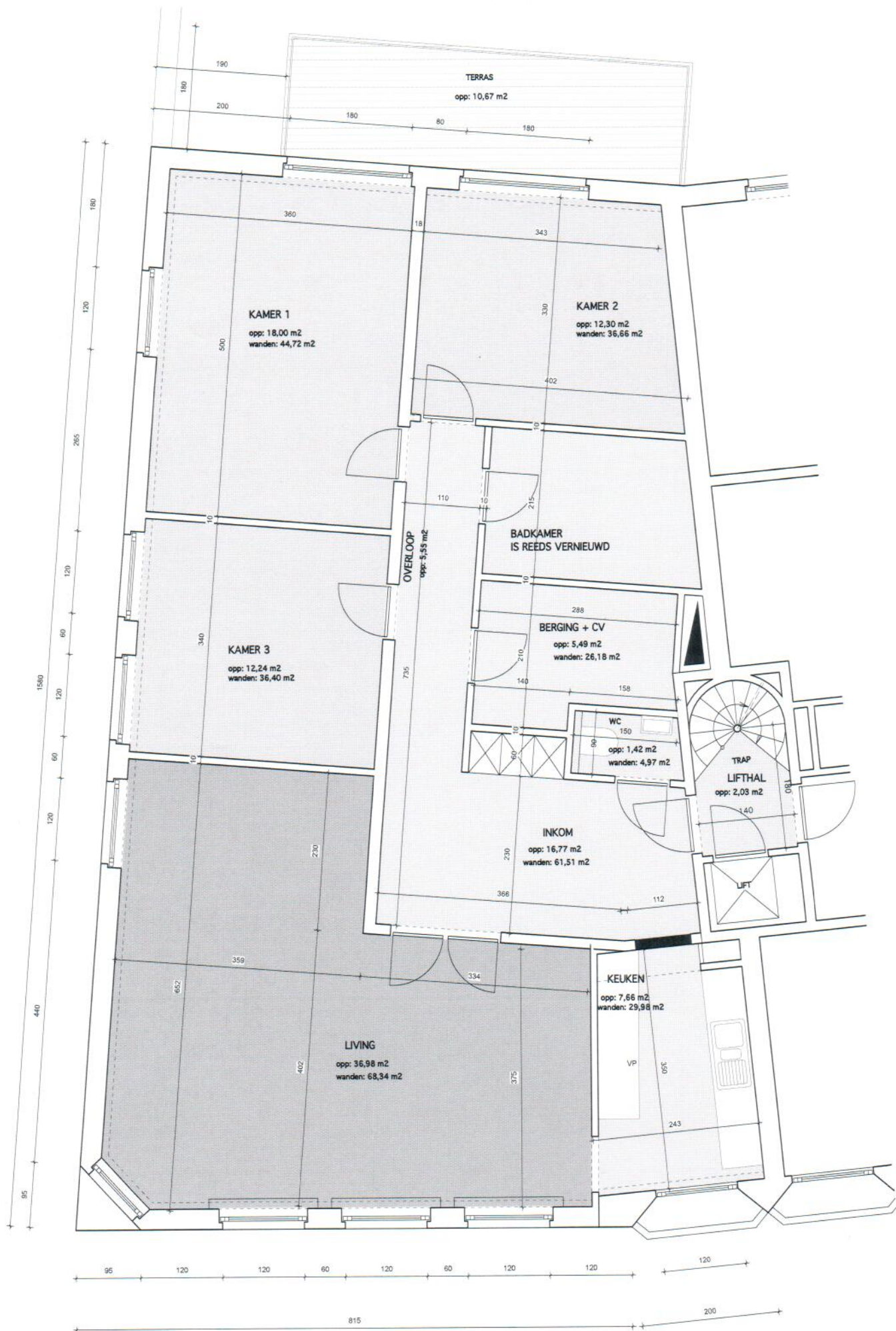
VERDIEPING 1 NIEUW 1/50
